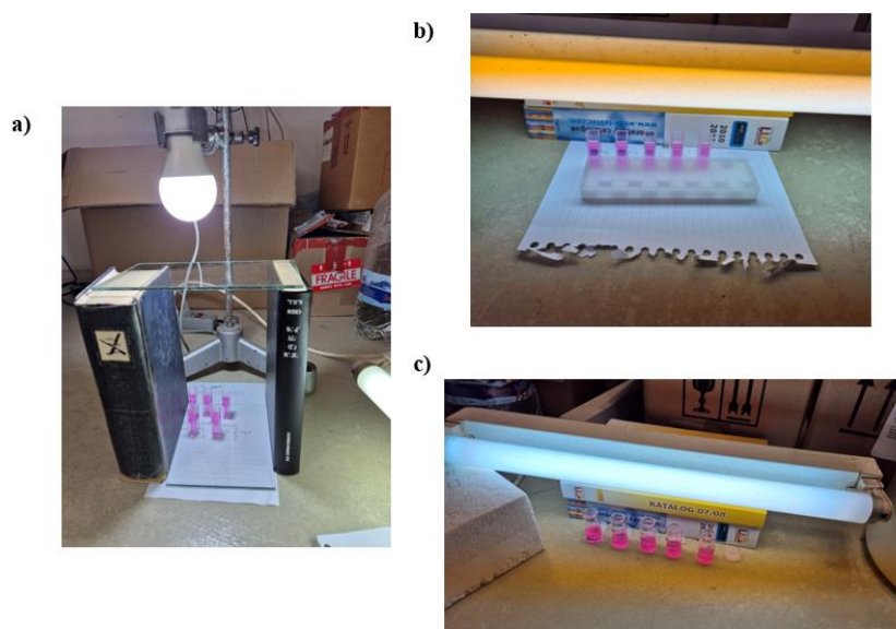
Slika 20. Analiza fotokatalitičke aktivnosti sintetiziranih HEO i \text{CeO}_2 korištenjem: a) izvora svijetla A b) izvora svjetla B c) izvora svjetla B uz dodatak kokatalizatora \text{H}_2\text{O}_2 .
