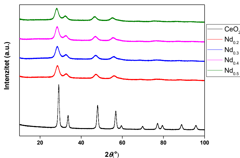
Slika 21. Preklapljeni difraktogrami sintetiziranih uzoraka s \text{CeO}_2 .
