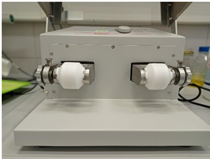
Slika 8. Vibracijski mlin.
