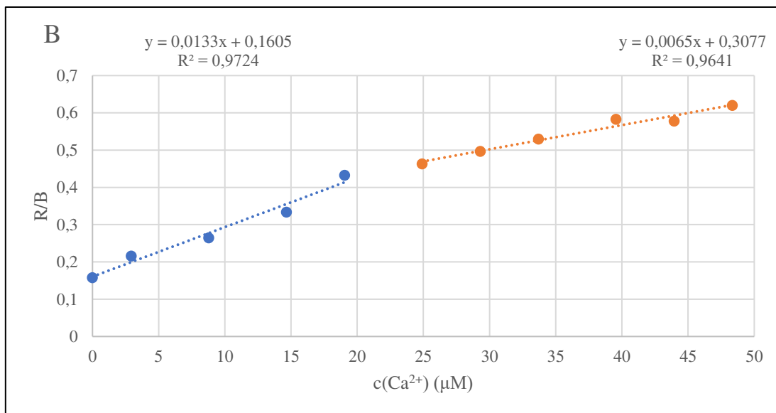
Slika 16. Ovisnost apsorbancije o koncentraciji Ca^{2+} u dva područja omjera analita i indikatora: A. 600 nm, B. 650 nm
