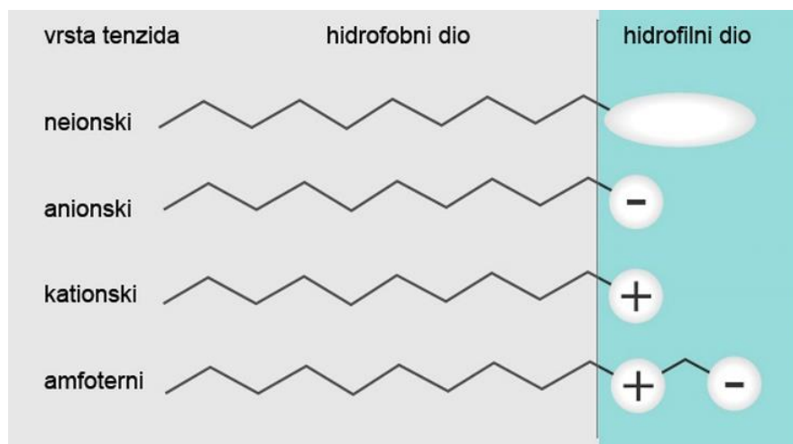
Slika 2. Klasifikacija tenzida [7].
