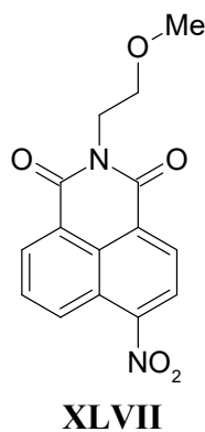
Slika 23. Strukturna formula molekule spoja XLVII [52]
