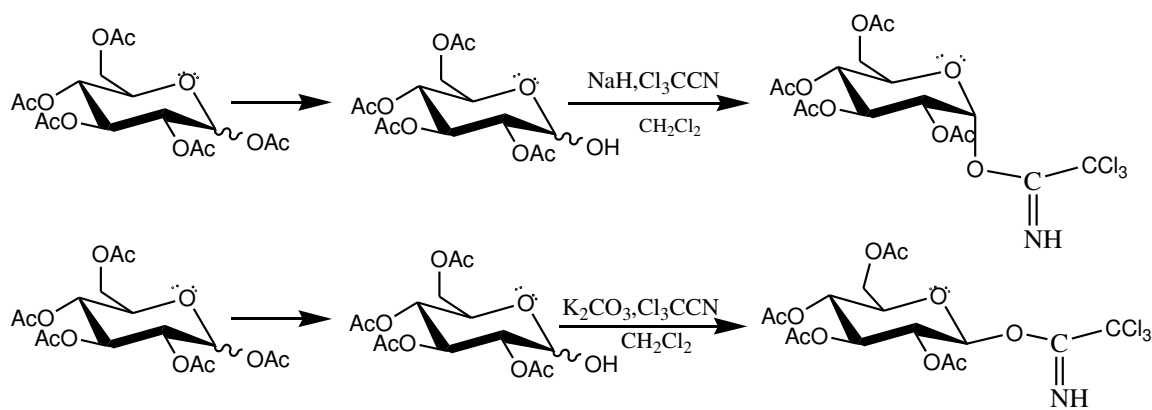
Slika 17. Sinteza glikozil-trikloroacetimidata
