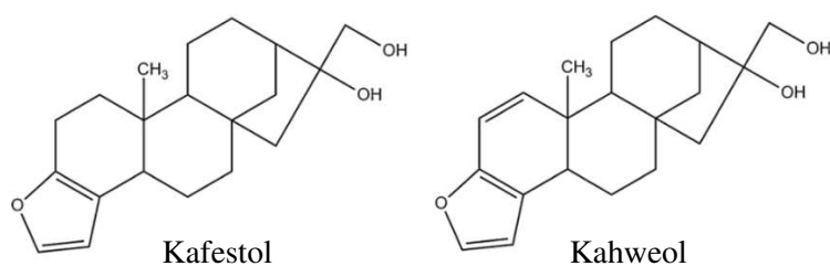
Slika 3. Kemijske strukture najznačajnijih terpena kave [19]
