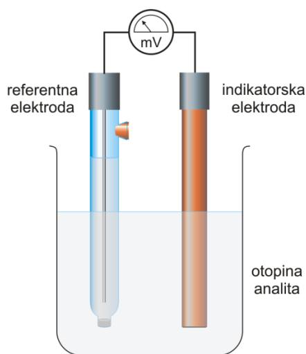
Slika 3. Elektrokemijska ćelija s elektrodnim parom [6]
